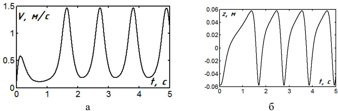
Рис. 4. Графіки зміни кінематичних параметрів при ковзанні частинки по еліпсу, який обертається із кутовою швидкістю \omega=20 \text{ с}^{-1} , при \beta=30^\circ , R=0,1 \text{ м} , f=f_R=0,3 : а) графік зміни відносної швидкості; б) графік зміни висоти відносного руху
