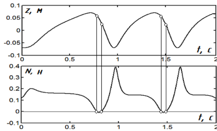
Рис. 6. Графіки зміни висоти z (вгорі) і реакції N площини (внизу) при \omega=24 \text{ c}^{-1} , \beta=35^\circ , R=0,1 \text{ м} , f=f_R=0,3
