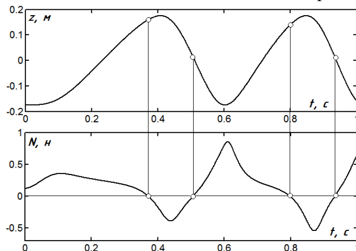
Рис. 7. Графіки зміни висоти z (вгорі) і реакції N площини (внизу) при \omega=24 \text{ c}^{-1} , \beta=35^\circ , R=0,25 \text{ м} , f=f_R=0,3
