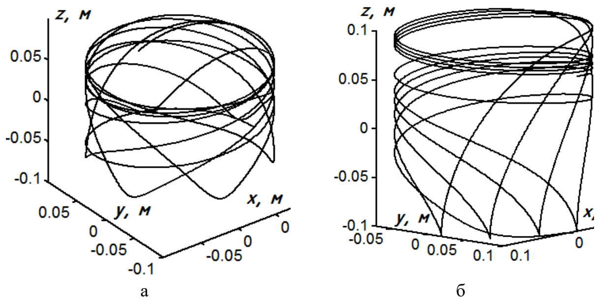
Рис. 8. Абсолютні траєкторії руху на внутрішній поверхні обмежувального циліндра радіуса R=0,1 : а) \omega=20 \text{ c}^{-1} , \beta=30^\circ , f=0,2 , f_R=0,3 ; б) \omega=18 \text{ c}^{-1} , \beta=45^\circ , f=0,1 , f_R=0,5
