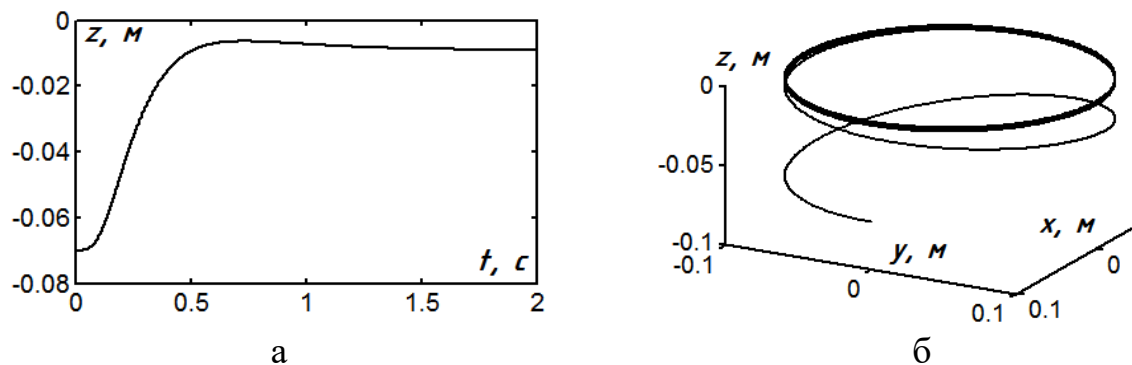
Рис. 5. Графіки зміни кінематичних параметрів при ковзанні частинки по еліпсу, який обертається із кутовою швидкістю \omega=20 \text{ с}^{-1} , при \beta=35^\circ , R=0,1 \text{ м} , f=f_R=0,3 : а) графік зміни висоти відносного руху; б) абсолютна траєкторія руху частинки
