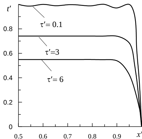
Рис. 2. Залежність безрозмірної температури t' від осової координати x' за різних значень часу ( \theta = 0 ; k = 1 ; Bi = 0.1 ).
