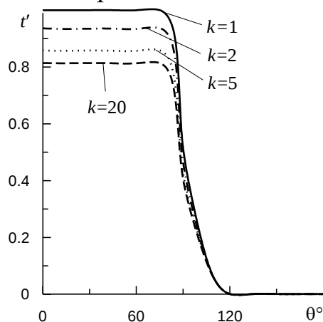
Рис. 1. Залежність безрозмірної температури t' від кутової координати \theta за різних значень коефіцієнта неоднорідності ( x' = 0.5; Bi = 0.1; \tau' = 0.1 ).
