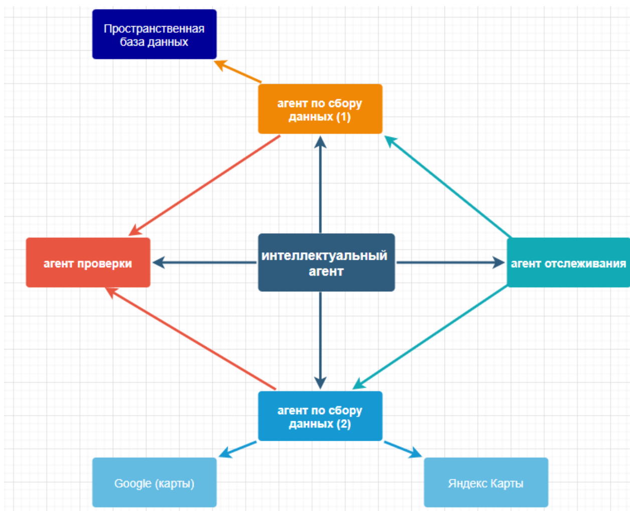
Рис. 1. Схема предложенной мультиагентной системы
